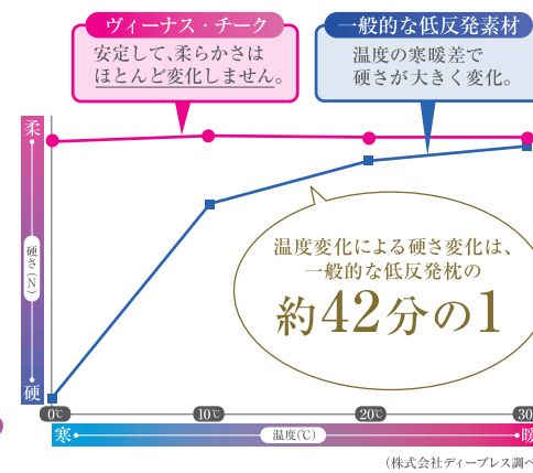
■温度依存性測定試験 湿度50%RHに保った状態で、圧力を加えて10mm沈め、枕から突き上げる圧力を0℃～30℃の温度下で測定した温度変化にともなう硬度の比較。
